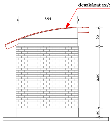
Oldalnézet
