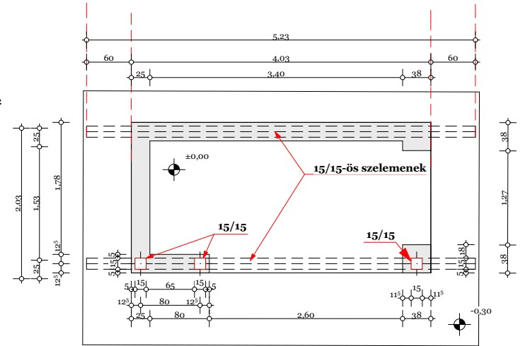
ALAPRAJZ
