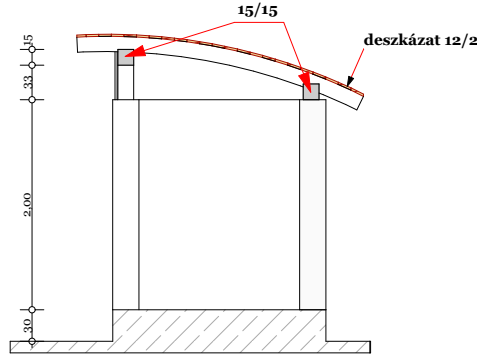
Oldalnézet
